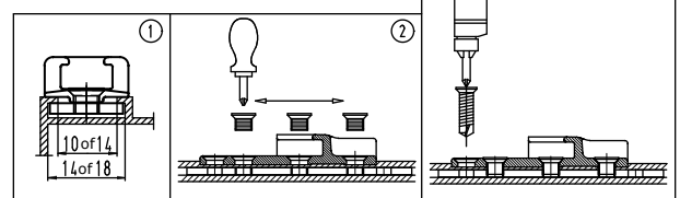
Plaatje inschuiven Plaatje aan sluitstuk vóór de montage vastschroeven Na positionering het sluitstuk vastschroeven
