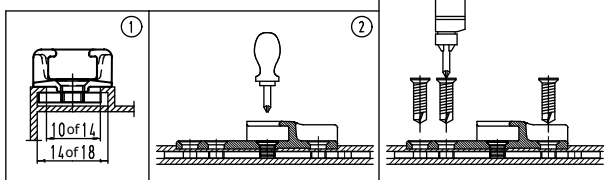
Sluitstuk inhaken Klem Schroef vastschroeven Na positionering het sluitstuk vastschroeven
