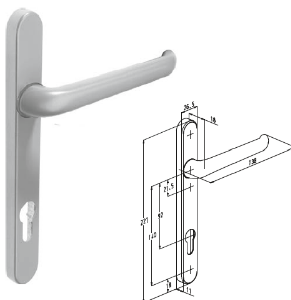
Rolluikkruk nr. 82002(C)L (binnenzijde) 82012(C)LVI (buitenzijde)
