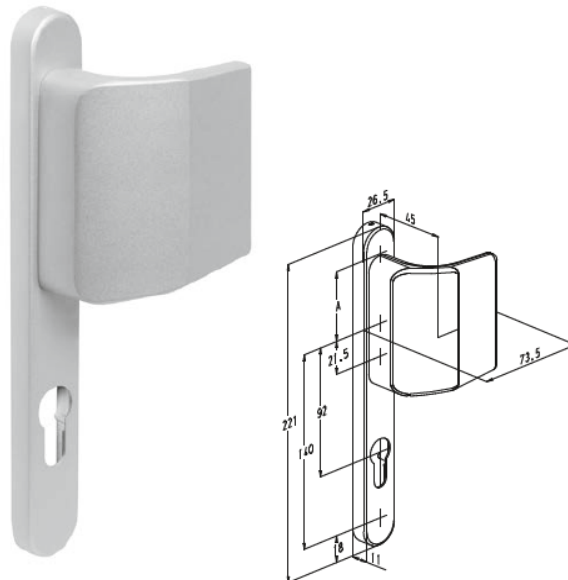
Deurtrekker nr. 82005(C)L (binnenzijde) 82015(C)LVI (buitenzijde)
